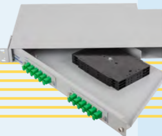
MCNP - Konnektör Panel Kabini
