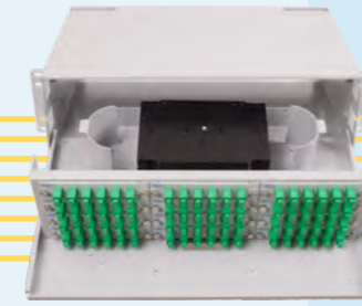
OFDU - Ekleme ve Sonlandırma Kabini
